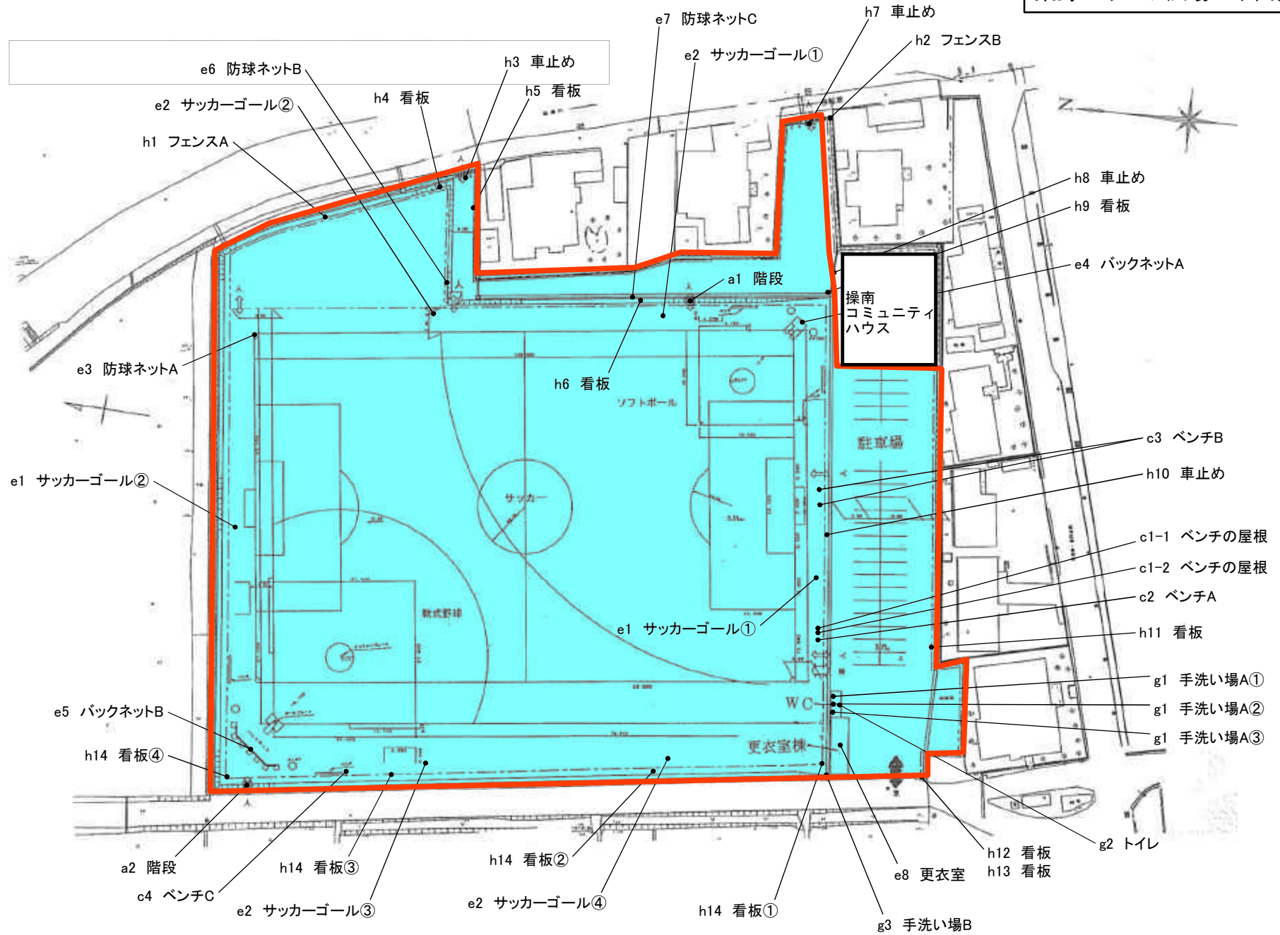
桑野スポーツ広場 平面図
