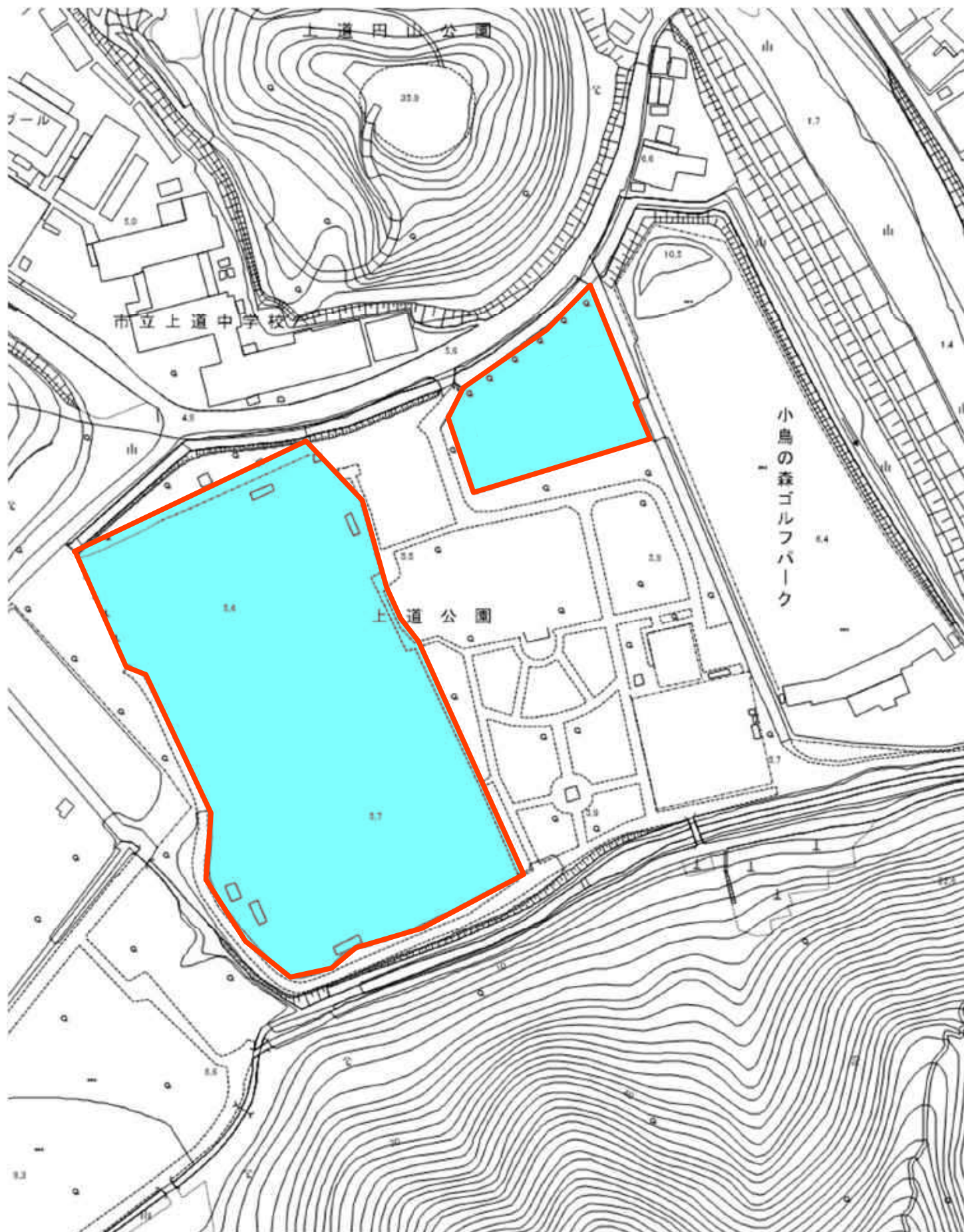
上道公園野球場 平面図
