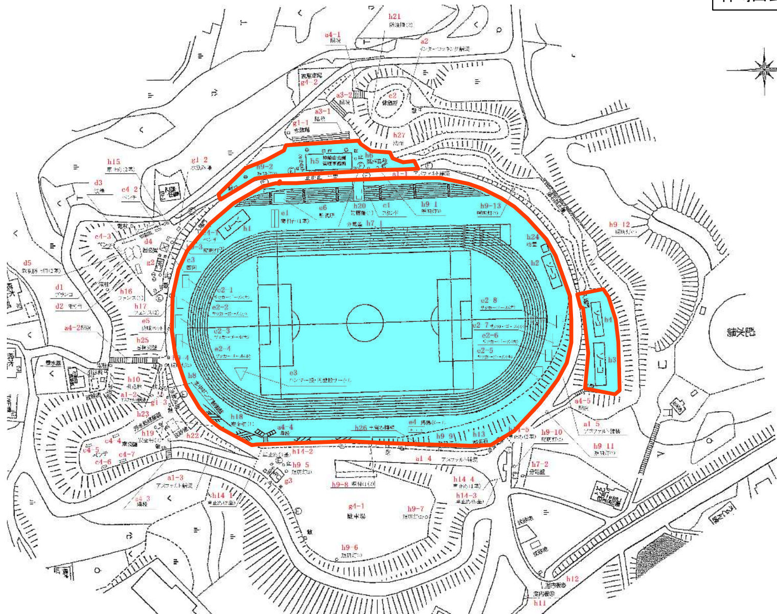
神崎山公園競技場 平面図
