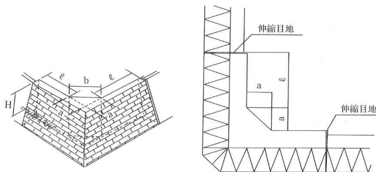
(a) 立体図
