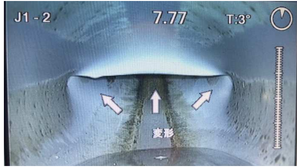
地震により変形した下水道管きよ
